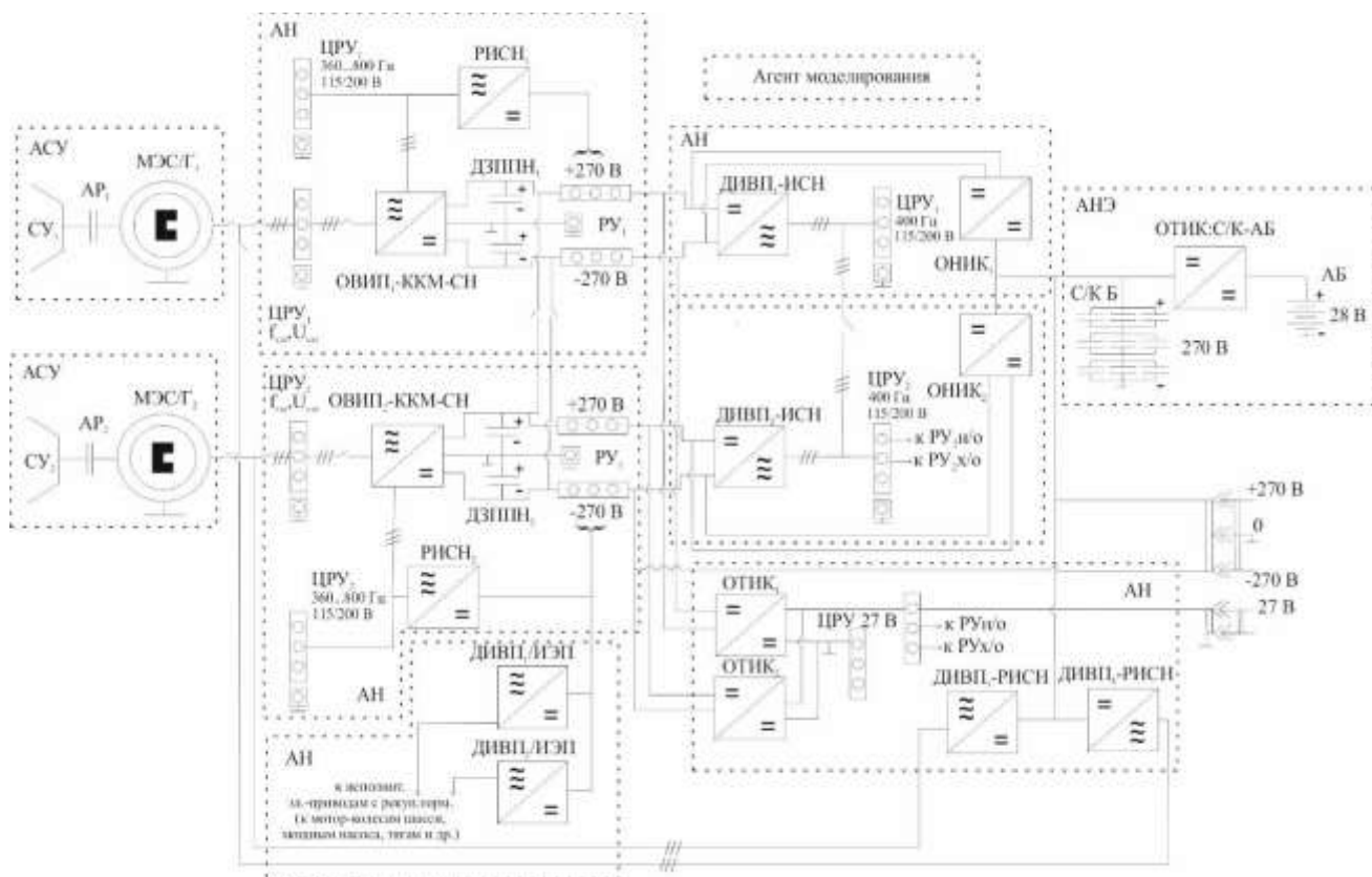
Рисунок 2. - Структурная схема ЭЭК БЭС с многоагентным подходом к управлению
