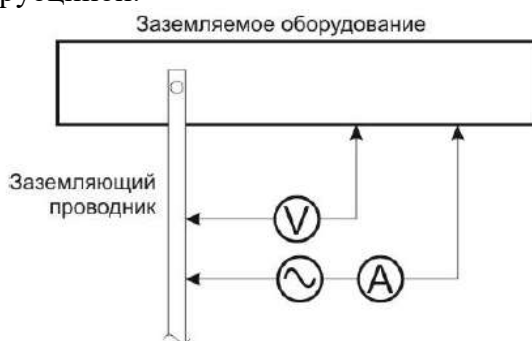
Рисунок 1 – Схема измерения сопротивления контактного соединений
