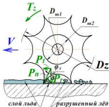
Рисунок 2 – Силевая схема разрушения ледового покрытия
