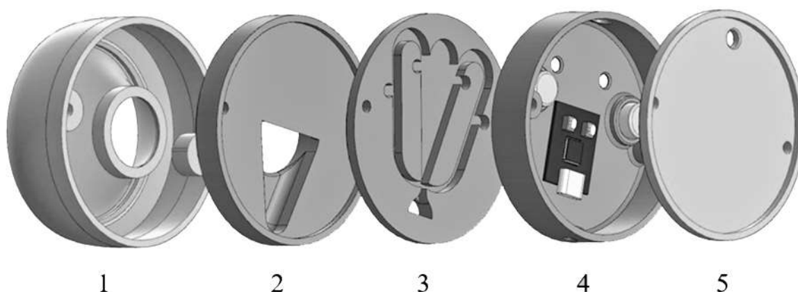
Рис. 2 – Основные элементы, составляющую конструкцию научного модуля:
