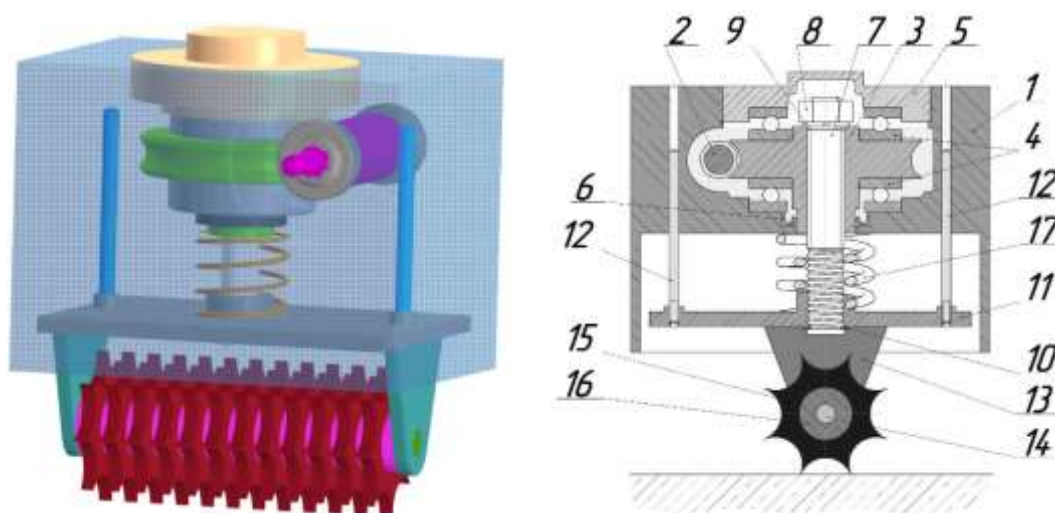
Рисунок 1 – Принципиальная схема устройства очистки снежно-ледовых масс с поверхности дорог
