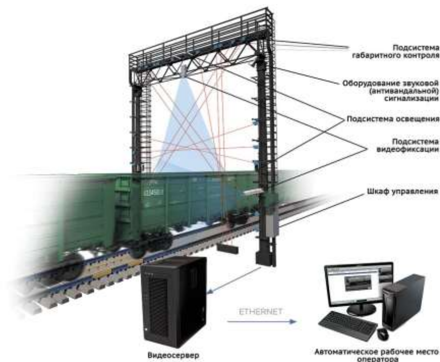
Рисунок 2 – Автоматизированная система коммерческого осмотра вагонов
