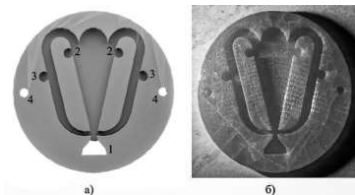
Рис. 1 – Функциональная плата струйного автогенератора:
