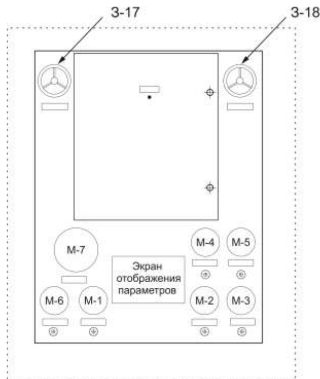
Рисунок 2 – Щит управления БРВ с контрольно-измерительными приборами запорными клапанами
