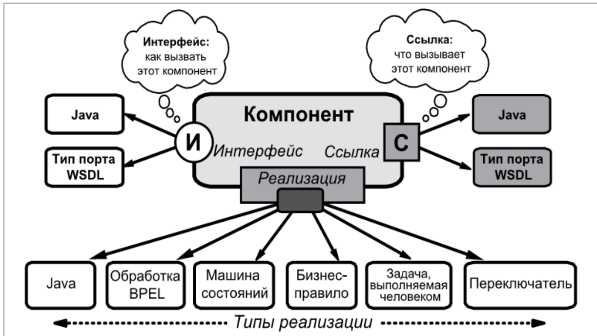
Рисунок 1 – Структура сервиса
