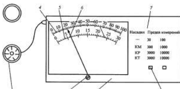
РИС. 1, 1-Корпус люкметра, 2-регулирующий винт, 3-фотоэлемент, 4- шкала с диапазоном измерений от 0 до 1000 лк, 5-шкала с диапазоном измерений от 0 до 300 лк, 6- стрелка указатель, 7 –таблица изменения диапазонов измерения в зависимости от применяемых насадок 8-переключатель диапазонов
